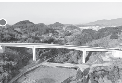
上部工/PC3径間ラーメン箱桁橋 下部工/逆T式橋台、柱式橋脚
